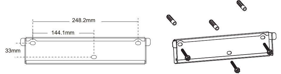
Fig. 2.1 Suporte de montagem na parede
