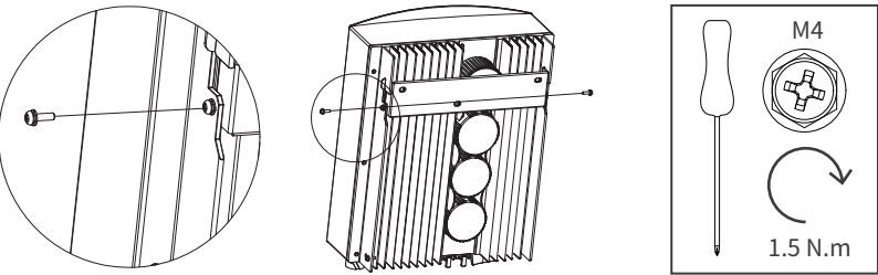
Fig. 2.3 Suporte de montagem na parede
