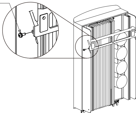
▲ Figura 4.5 Suporte de montagem em parede
