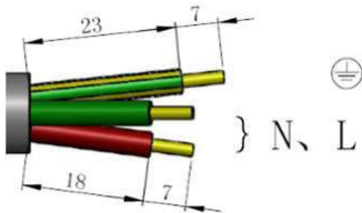
▲ Figura 4.15 Fios CA descarnados
