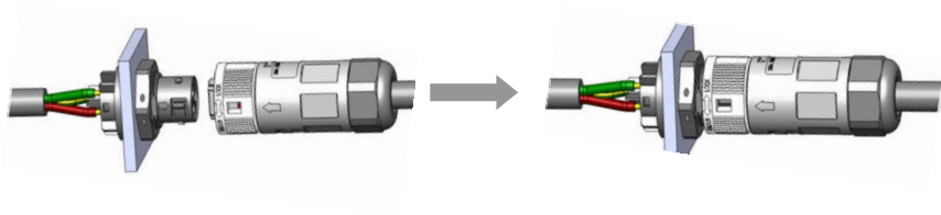
▲ Figura 4.18 Conecte o Conector AC Ao Inverter
