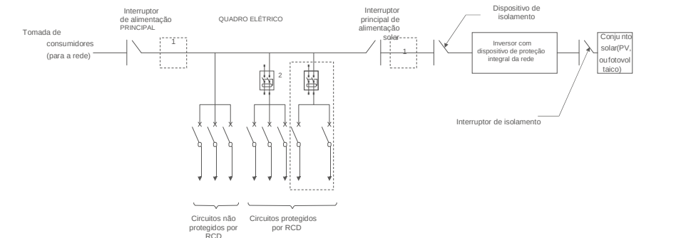
▲ Figura 4.21 Orientação para uma instalação simples de um sistema inversor de energia solar 1. O RCD deve estar em ligação paralela entre a rede do consumidor e o fornecimento solar. 2. Mais de um RCD pode ser usado. Cada RCD pode proteger um ou mais circuitos.
