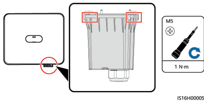
Figura 4-10 Instalação da caixa de junção
