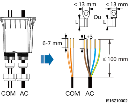
Figura 5-8 Passagem dos cabos
