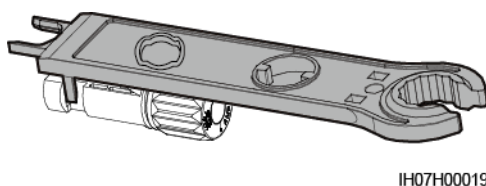
Figura 5-6 Remoção de um conector CC
