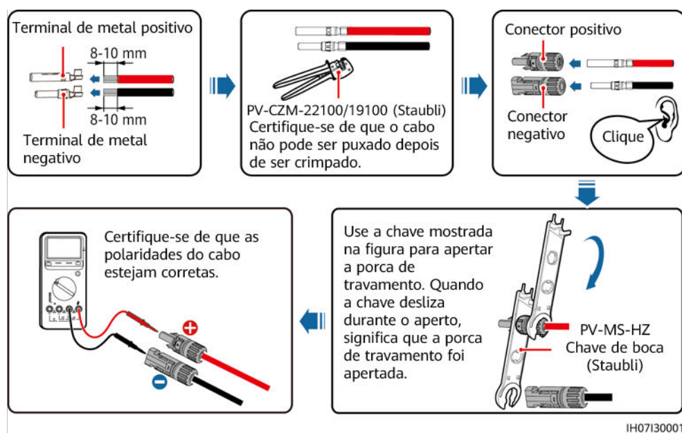
Figura 5-5 Montagem dos conectores CC
