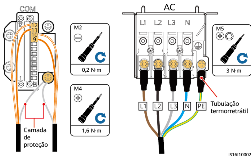
Figura 5-9 Instalação dos cabos de alimentação de saída CA e cabos de sinal
