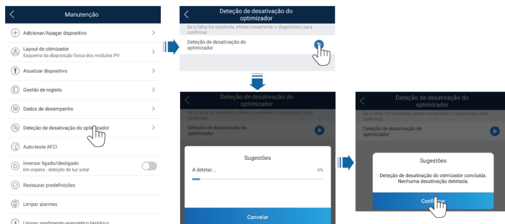
Figura 7-6 Detecte a desconexão do otimizador
