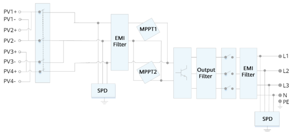
Figura 2-6 Diagrama conceitual
