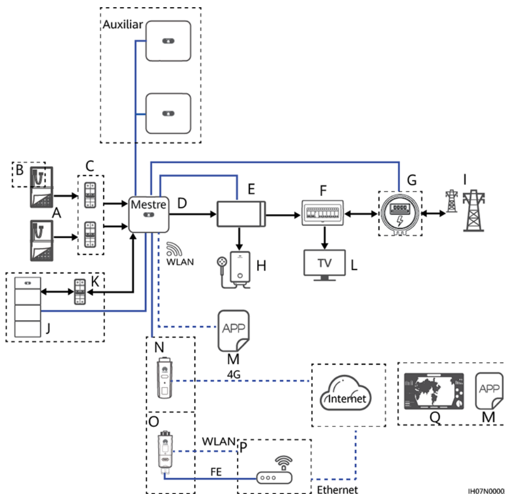
Figura 2-3 Cenário em cascata do SUN2000 (as caixas tracejadas indicam configuração opcional)
